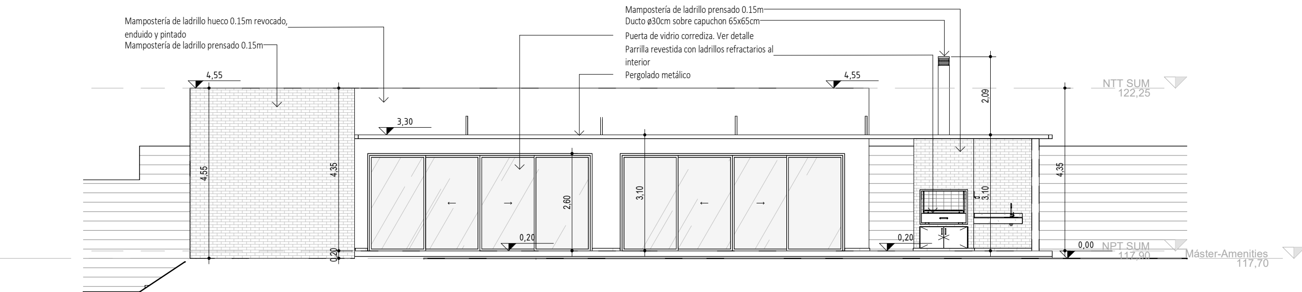
Fachada - SUM ESCALA 1:100
