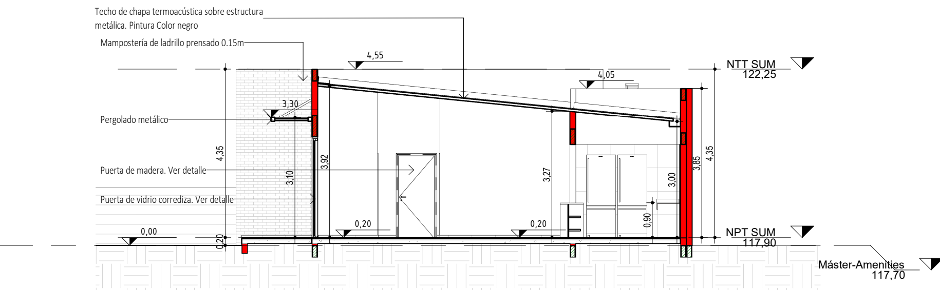
Corte A ESCALA 1:100
