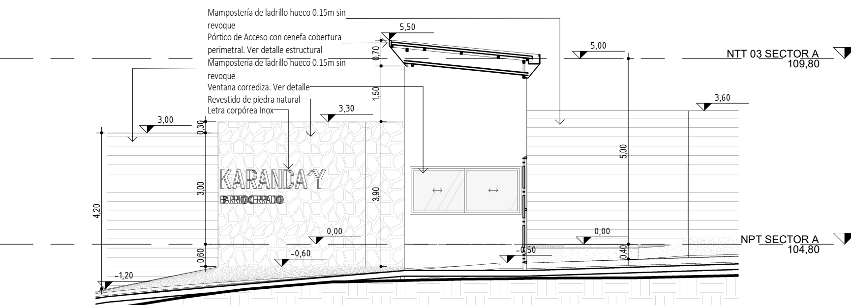
Corte C ESCALA 1:100
