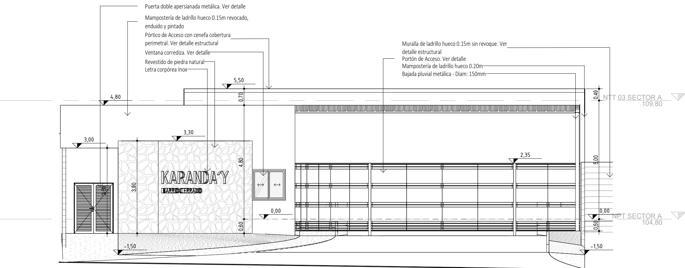
Fachada - Acceso 1 ESCALA 1:100
