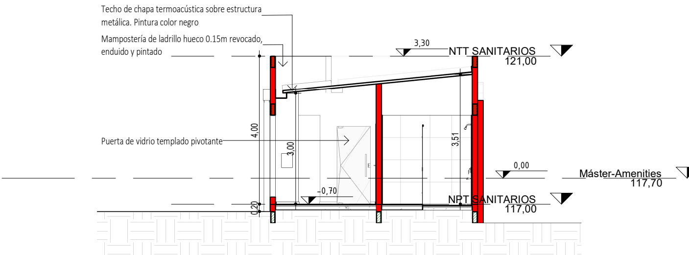
Corte B ESCALA 1:100
